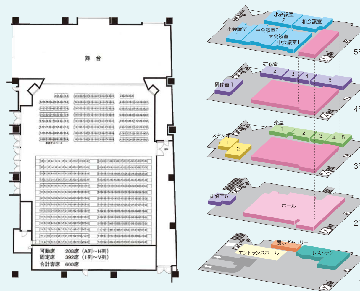
2F ホール（最大の客席パターン）
